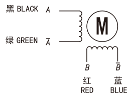
电机接线图
